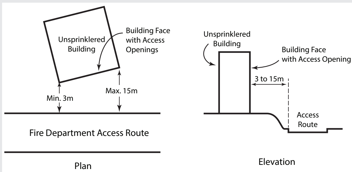
Figure A-3.2.5.5.-A
